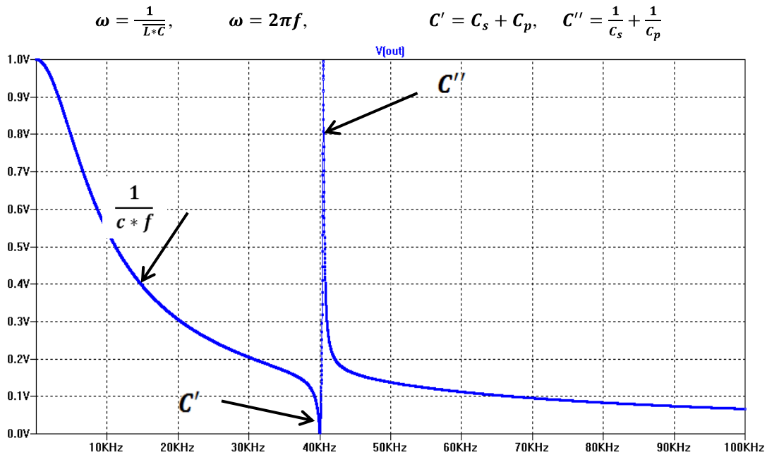
Рис. 2. АЧХ ультразвукового элемента
