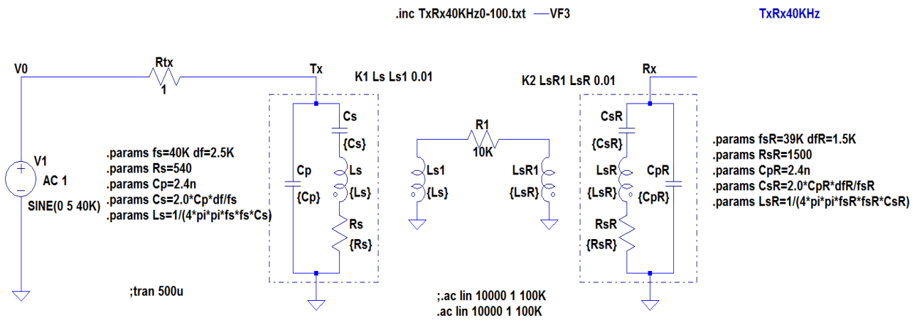
Рис. 8. LT-spice-модель акустической связи электроакустических элементов
